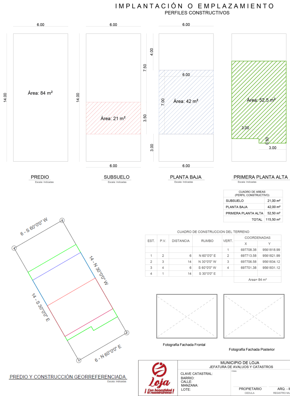
Figura 3: Plano del perfil constructivo.
