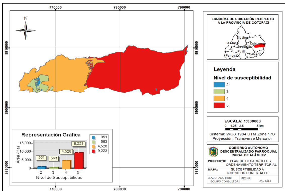
Mapa 19: Susceptibilidad a incendios forestales
