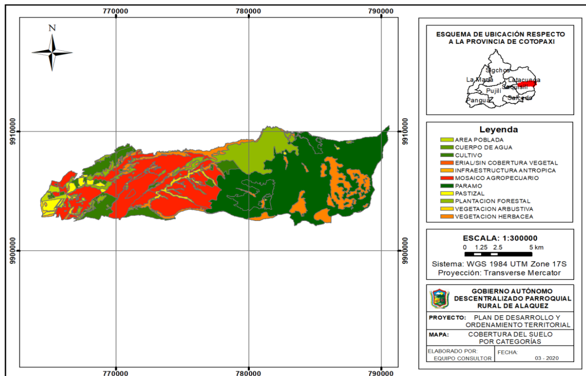
Mapa 15.- Cobertura del suelo por categorías
