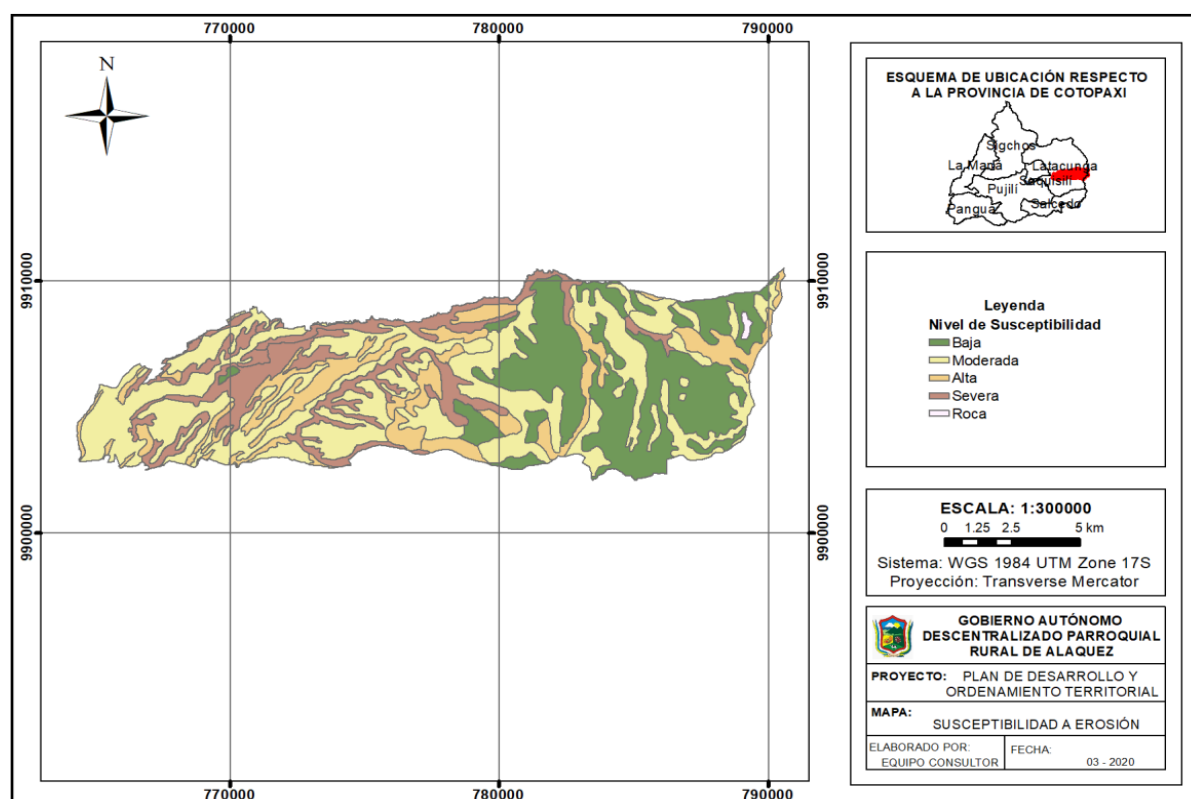
Mapa 12: Susceptibilidad a Erosión
