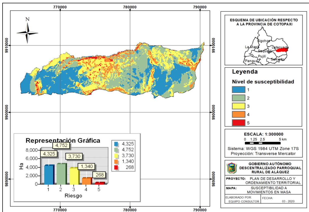
Mapa 20.- Susceptibilidad a movimientos en masa
