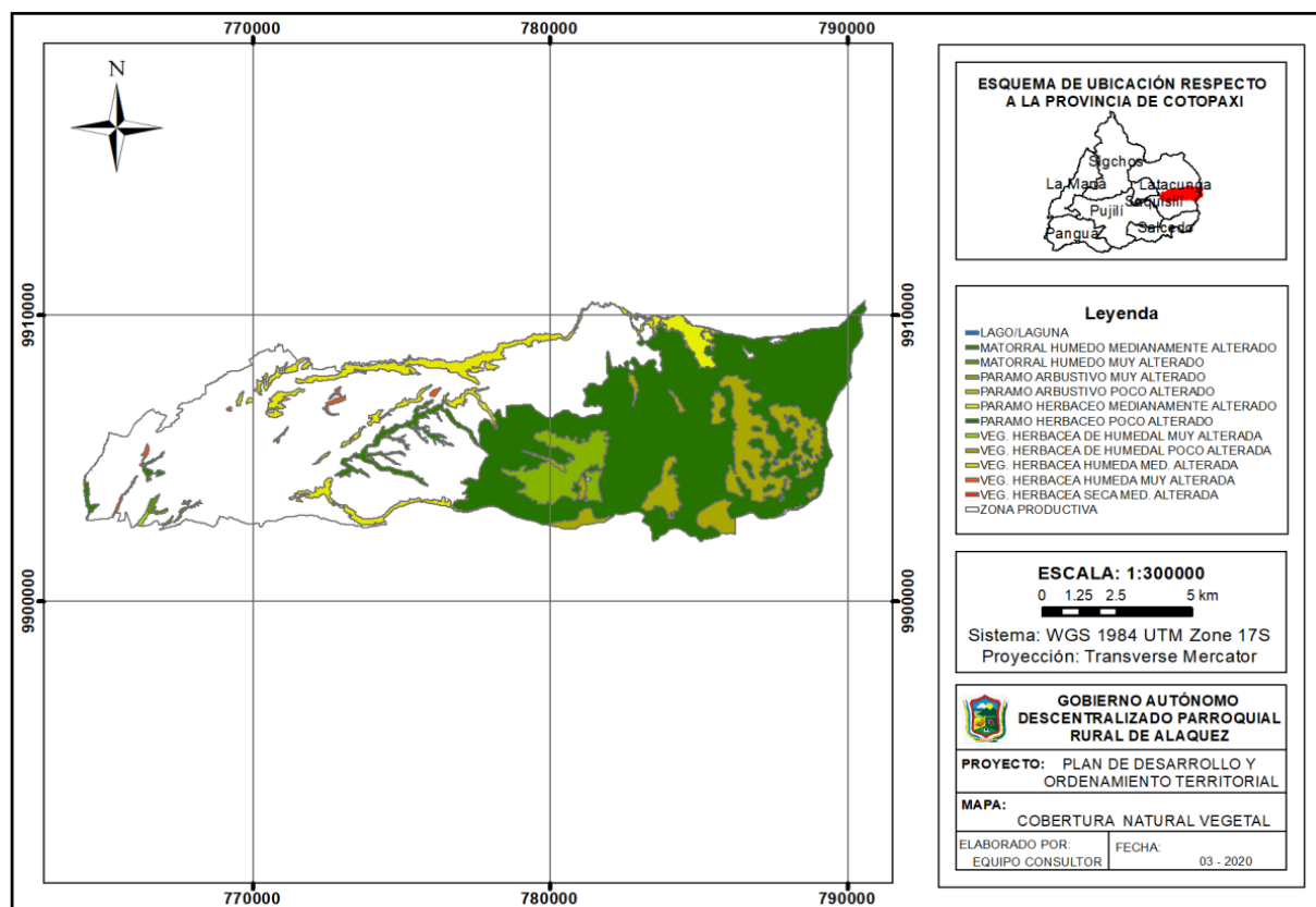
Mapa 14.- Cobertura natural vegetal
