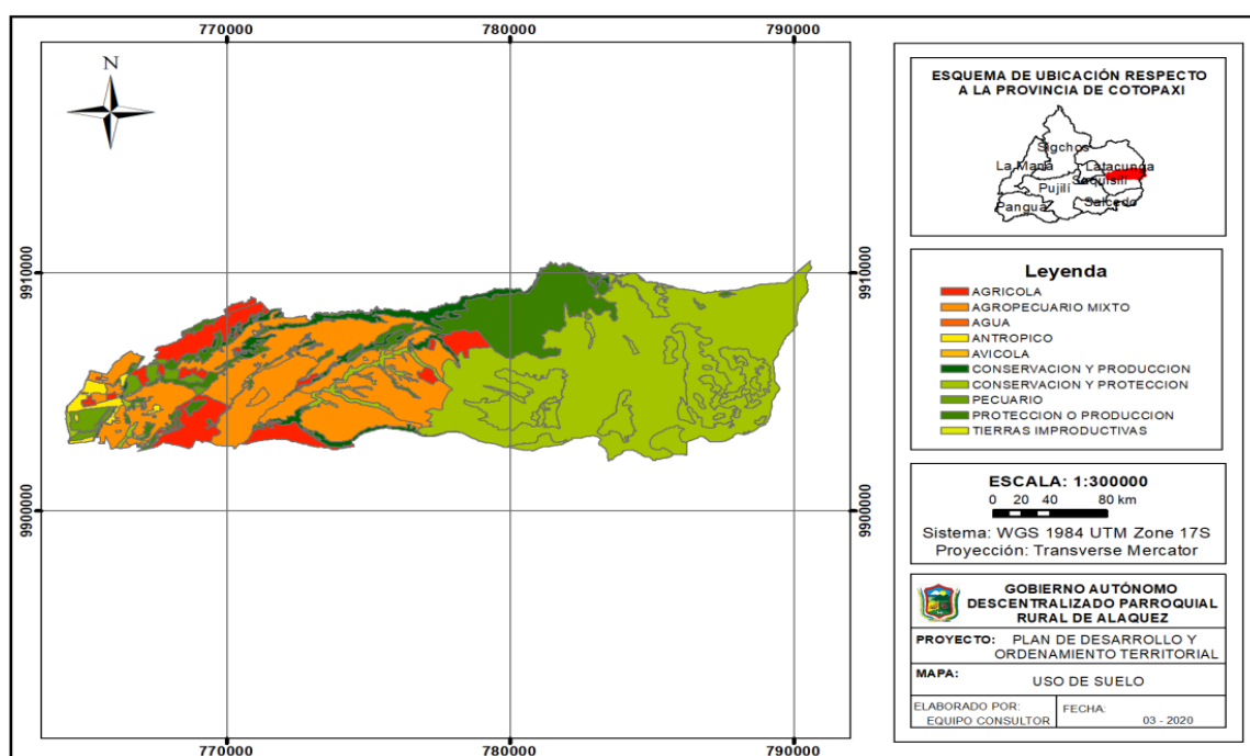
Mapa 16.- Uso del suelo
