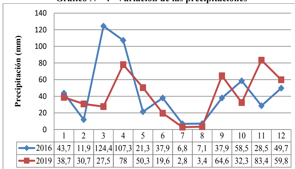
Gráfico N° 4 Variación de las precipitaciones
