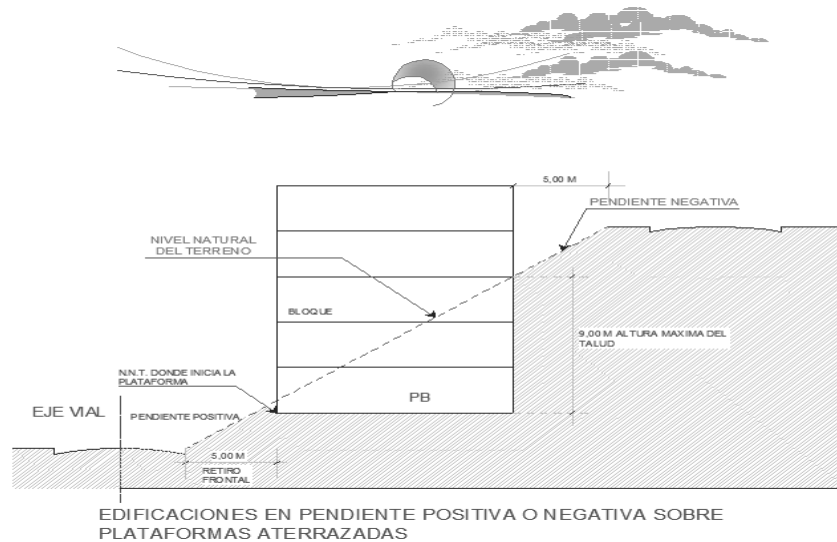
Gráfico No. 6: Edificaciones en Pendiente Positiva o Negativa sobre Plataformas Aterrazadas
