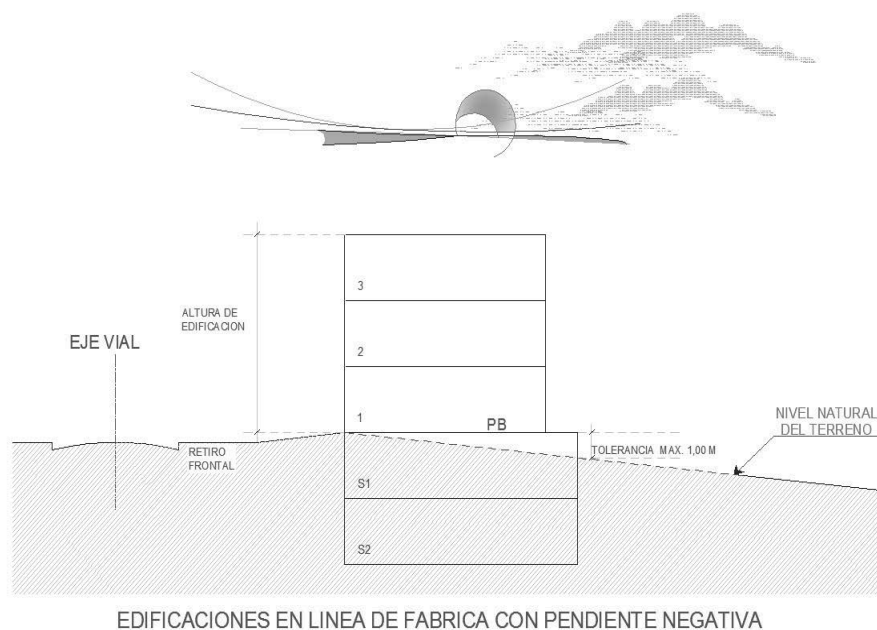
Gráfico No. 6b: Edificaciones sobre plataformas aterrazadas: en línea de fábrica con pendiente negativa
