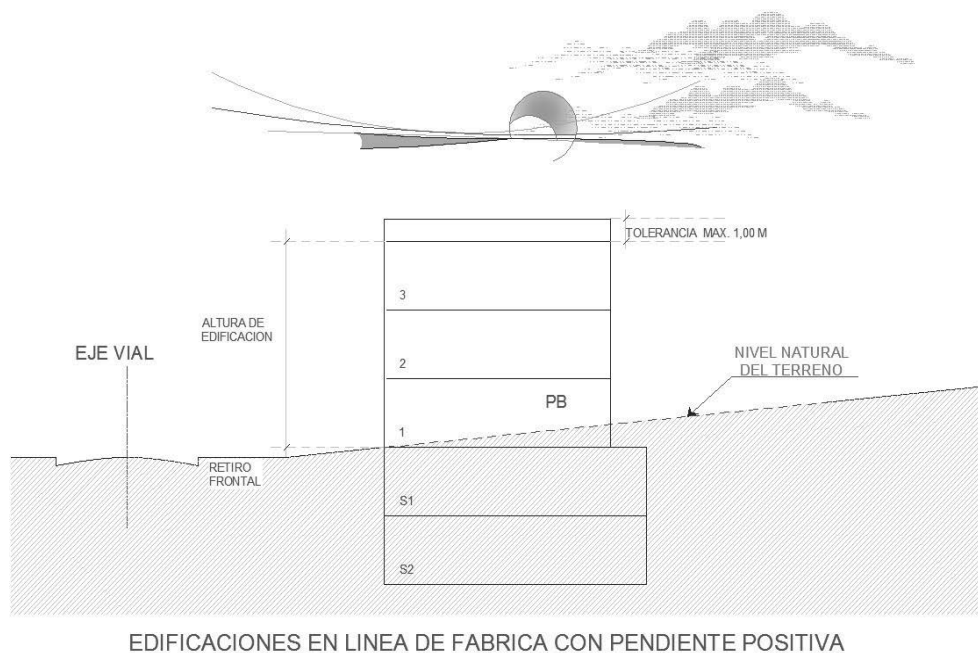
Gráfico No. 6a: Edificaciones sobre Plataformas Aterrazadas: en línea de fábrica con pendiente positiva
