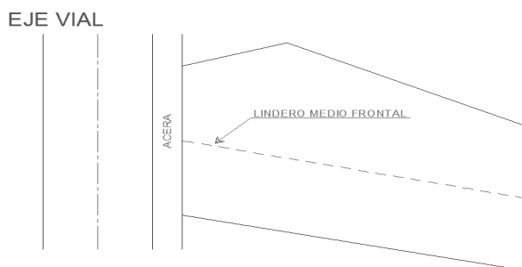
Gráfico No. 3: Pendientes referencial en terrenos irregulares
