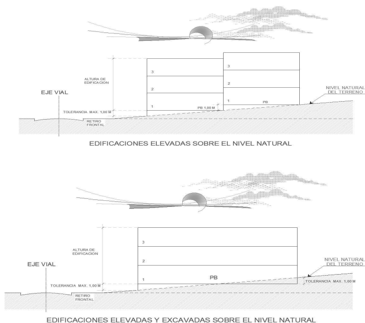
Gráfico No. 5a y Gráfico No. 5b: Edificaciones excavadas sobre nivel natural
