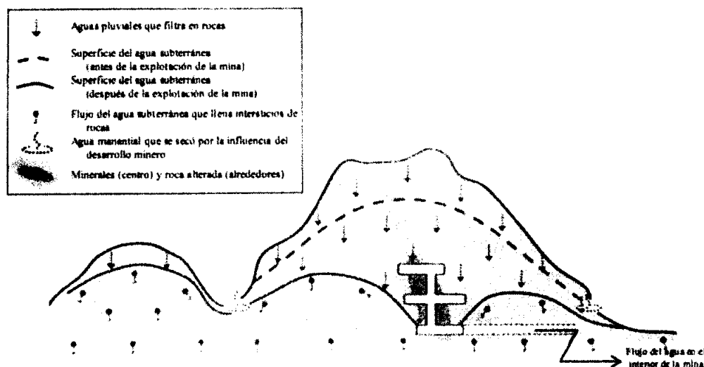
Fig. 4: Esquema de alteración del flujo de agua por la mina subterránea (JOCMEC 4)
