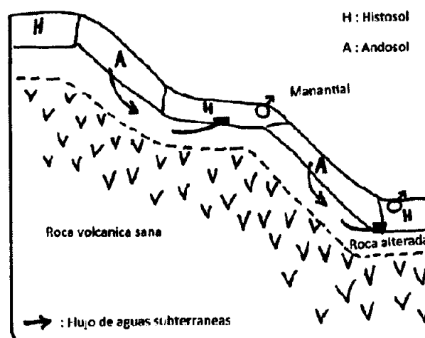
Fig. 3: modelo conceptual de circulación subterránea en Loma Larga (Fuente BRGM 2 )
