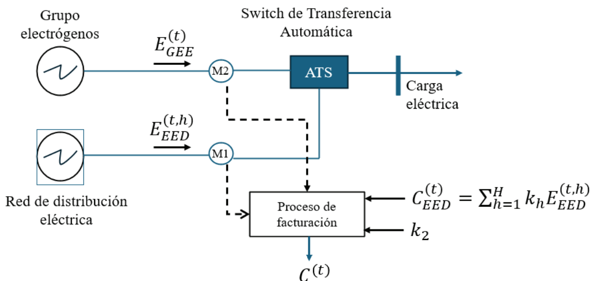
Figura 1 Esquema unifilar y diagrama de flujo de información para el modelo de facturación con generación de los GEE
