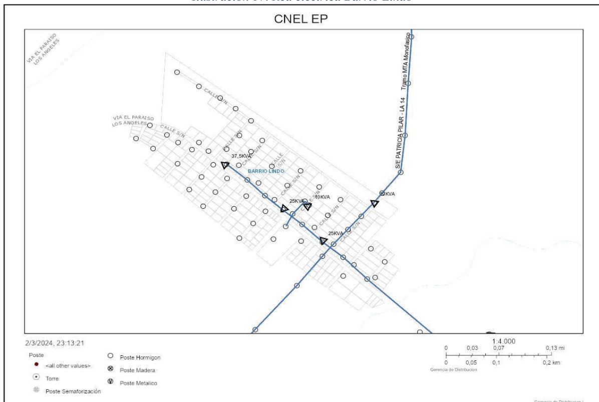
Ilustración 17. Red eléctrica Barrio Lindo
