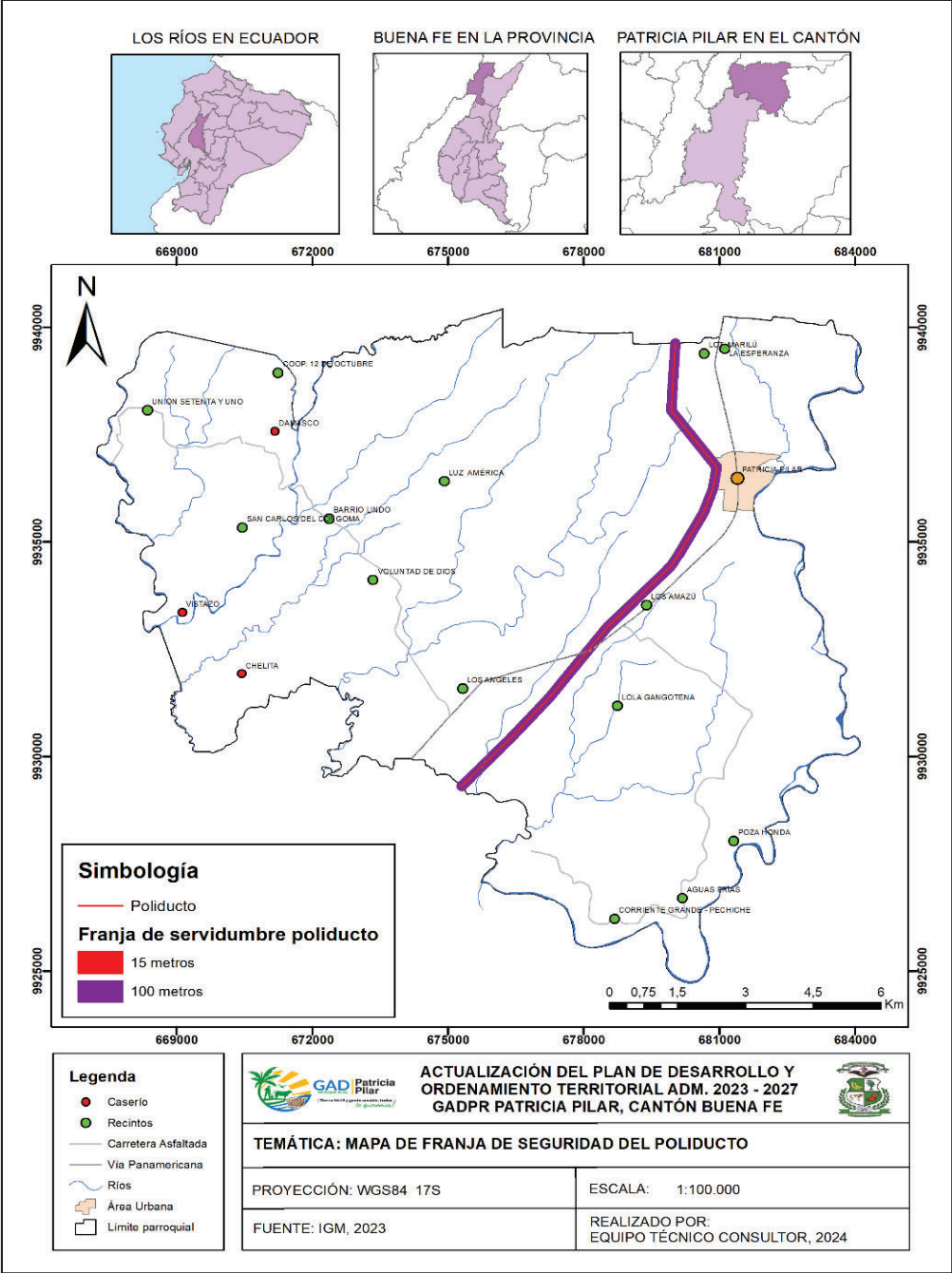
Mapa 33. Franja de seguridad del poliducto
