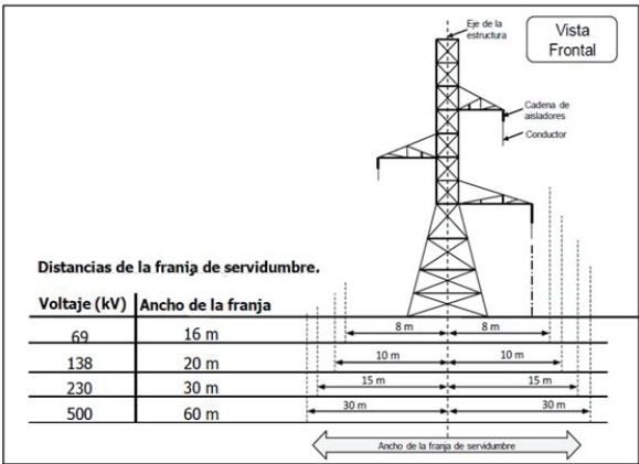
Ilustración 46. Franja de protección de las líneas transmisión eléctrica
