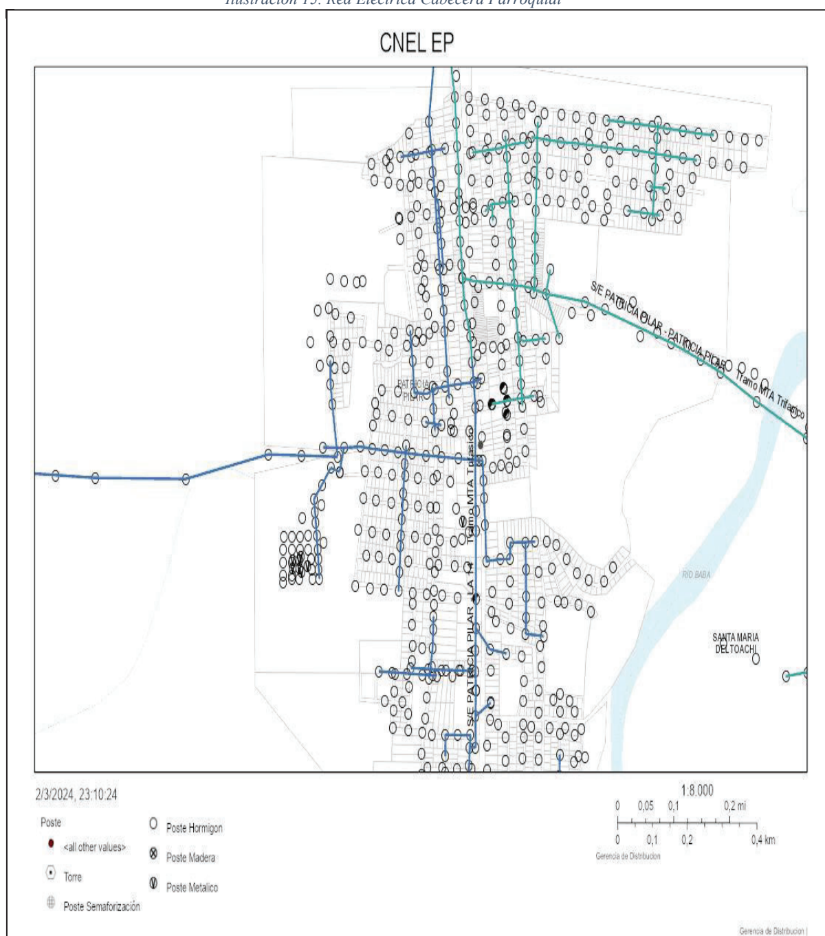
Ilustración 15. Red Eléctrica Cabecera Parroquial
