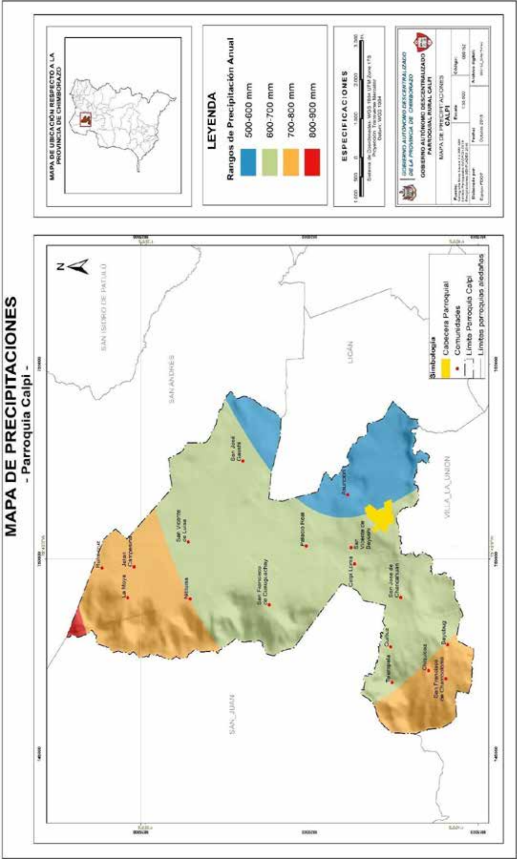
Mapa N3 3 Precipitaciones
