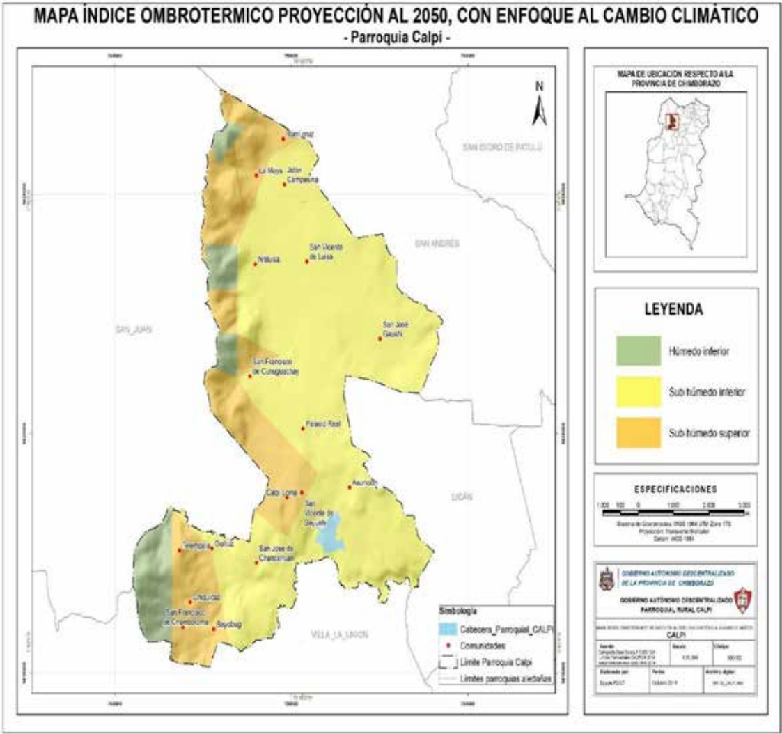
Mapa N° 5 Índice ombrotérmico – proyección al 2050, con enfoque al cambio climático
