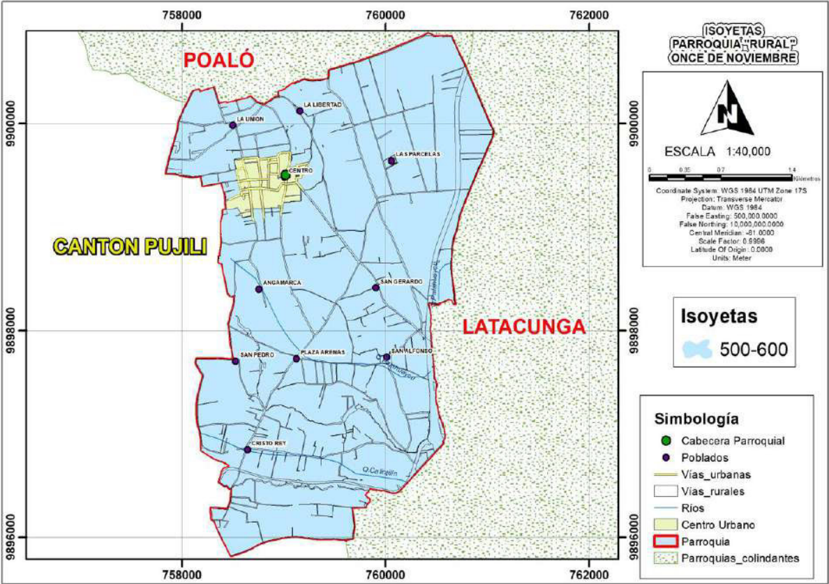
Mapa 12. Isoyetas.
