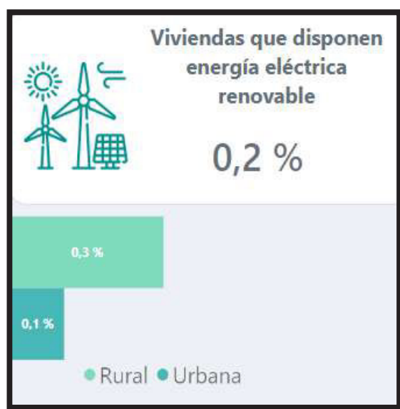
Gráfico 26. Energías renovables.
