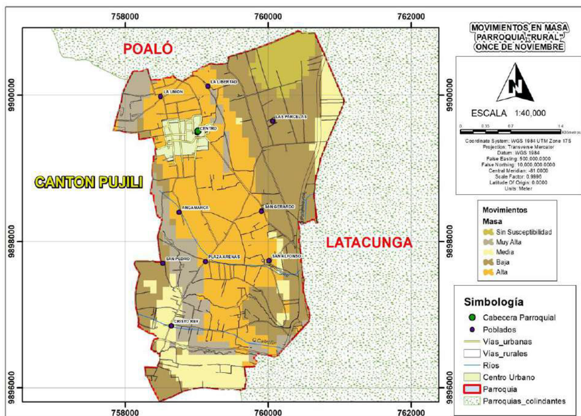
Mapa 6. Movimientos en masa.
