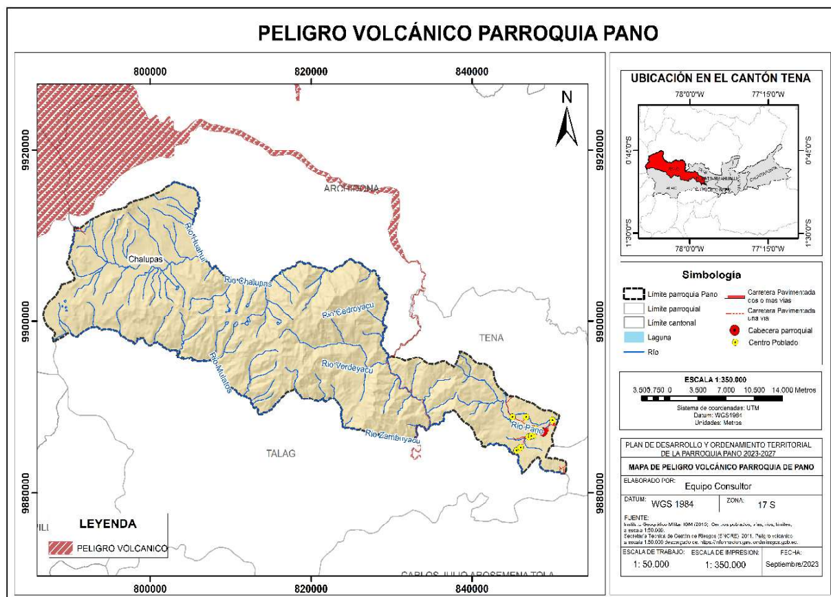
Mapa 15 Peligro volcánico
