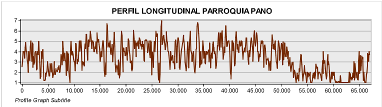
Figura 1. Perfil longitudinal
