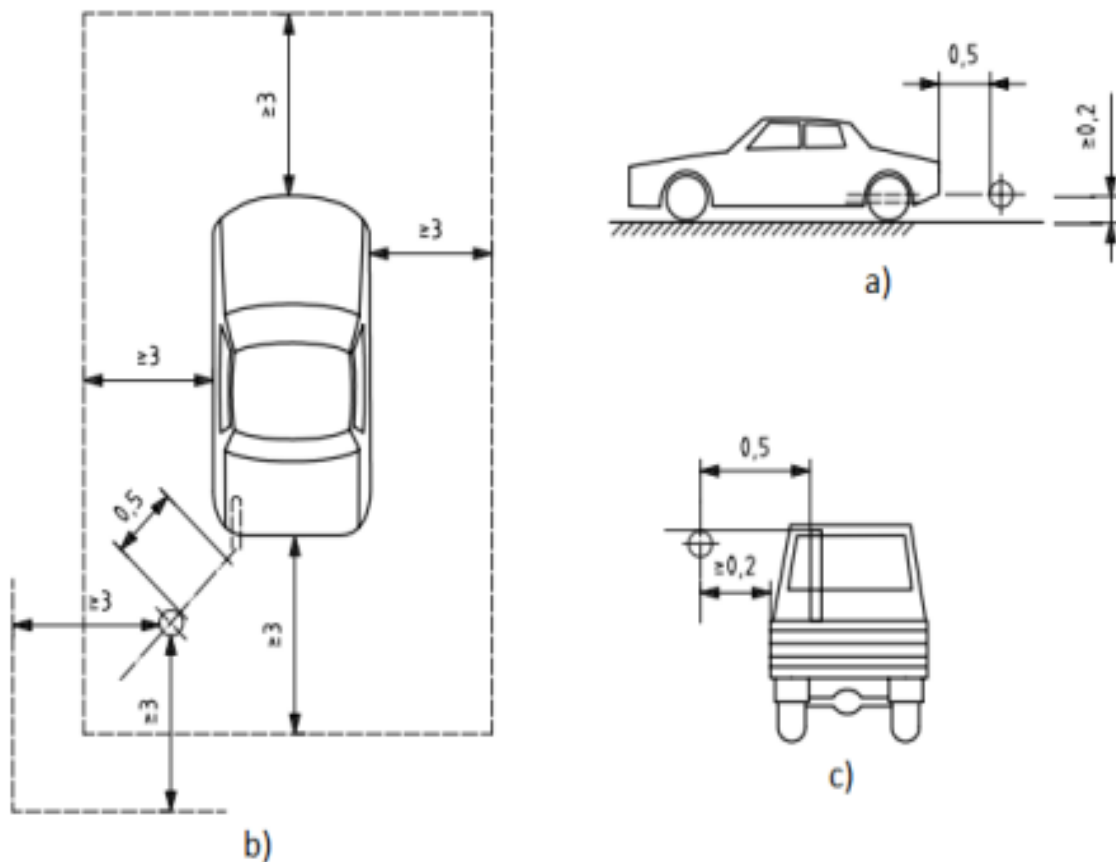
Figura 1. MEDICIÓN DE RUIDO PARA FMR. Fuente: ISO 5130:2007
