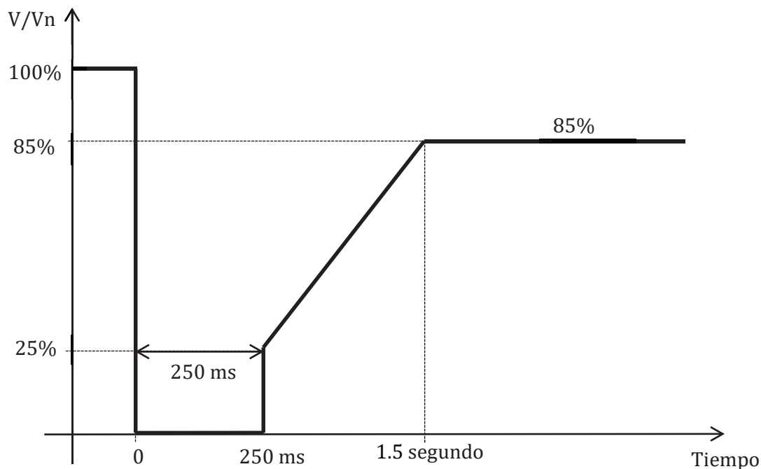
Gráfico 8 Perfil de la Capacidad para Soportar Huecos de Voltaje de una Unidad de Generación Síncrona o Unidad de Parque Eléctrico categoría D
