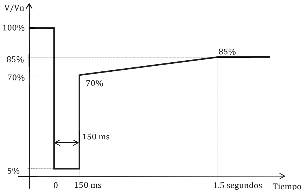
Gráfico 3 Perfil de la Capacidad para Soportar Huecos de Voltaje de una Central de Generación síncrona.
