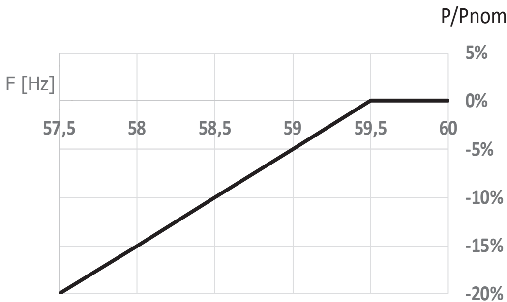
Gráfico 2 Reducción de capacidad de la Potencia Nominal ante una caída de la Frecuencia.
