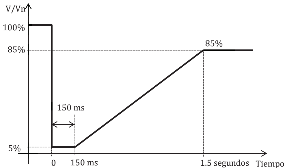
Gráfico 4 Perfil de la Capacidad para Soportar Huecos de Voltaje de una Unidad de Parque Eléctrico
