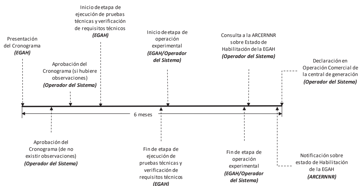
Ilustración 2 Proceso para aprobación de cronograma y ejecución de Pruebas Técnicas y Operación Experimental, previas a la Declaración en Operación Comercial de Centrales o Unidades de Generación categorías B, C o D.
