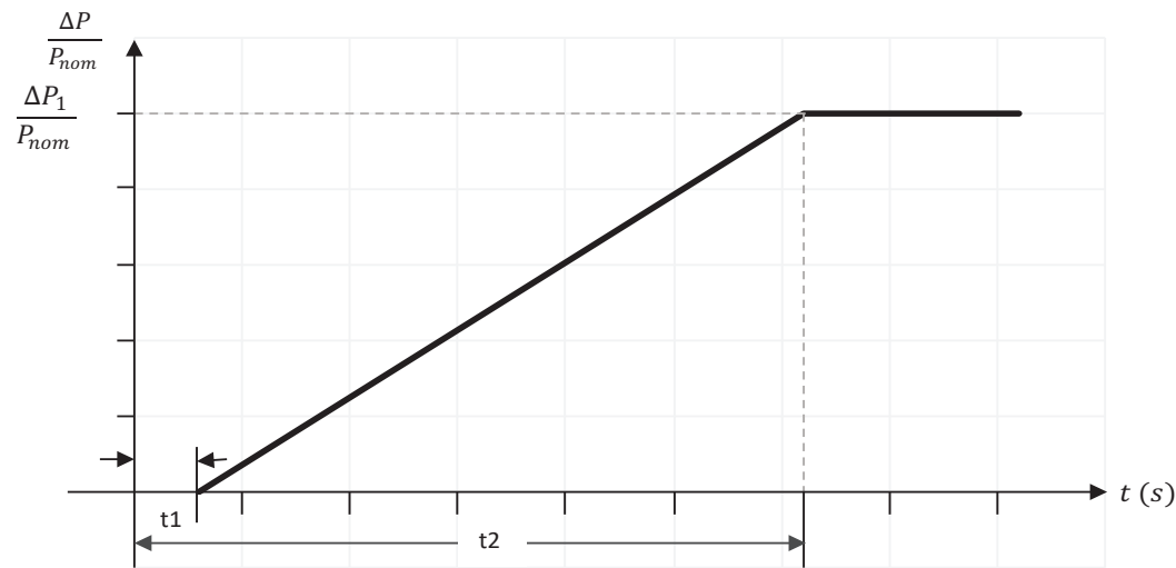
Gráfico 6 Capacidad de respuesta de la Potencia Activa ante variaciones de Frecuencia
