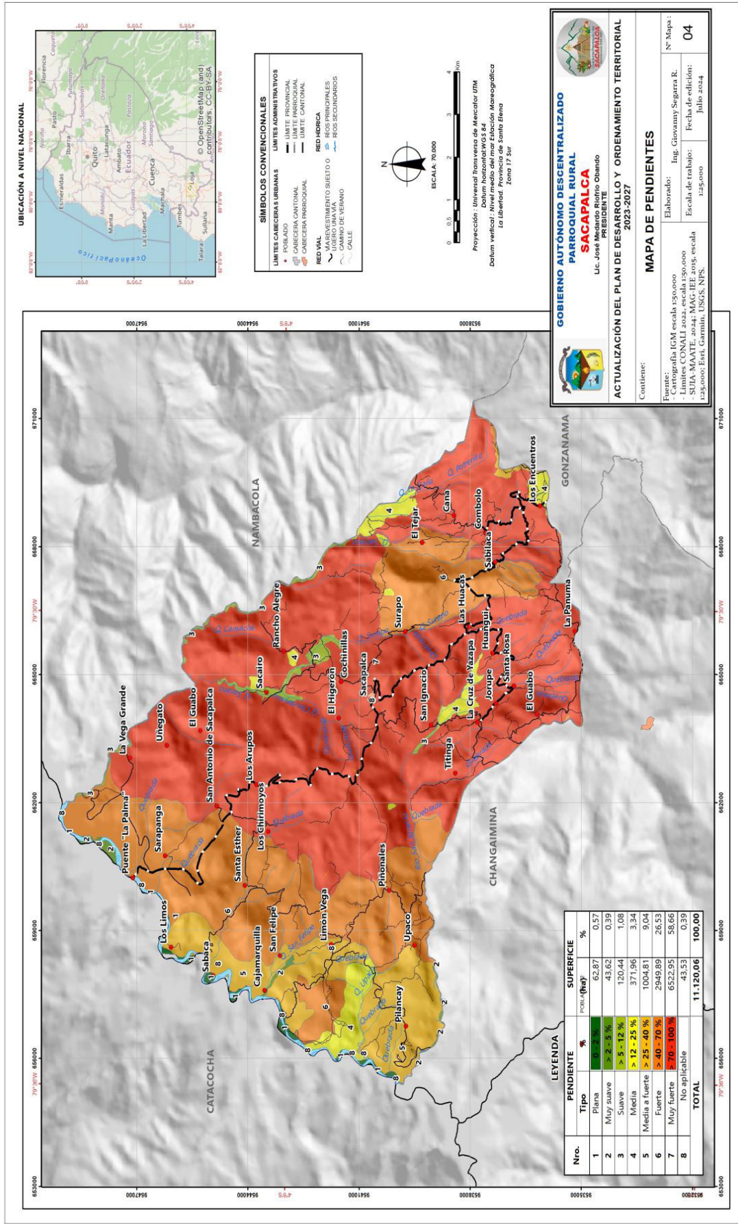
Mapa 10. Pendientes - Parroquia Sacapalca
