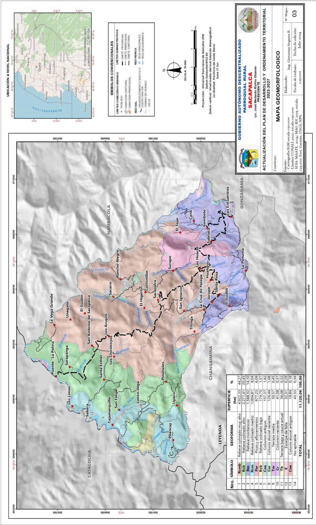
Mapa 8. Geomorfología - Parroquia Sacapalca
