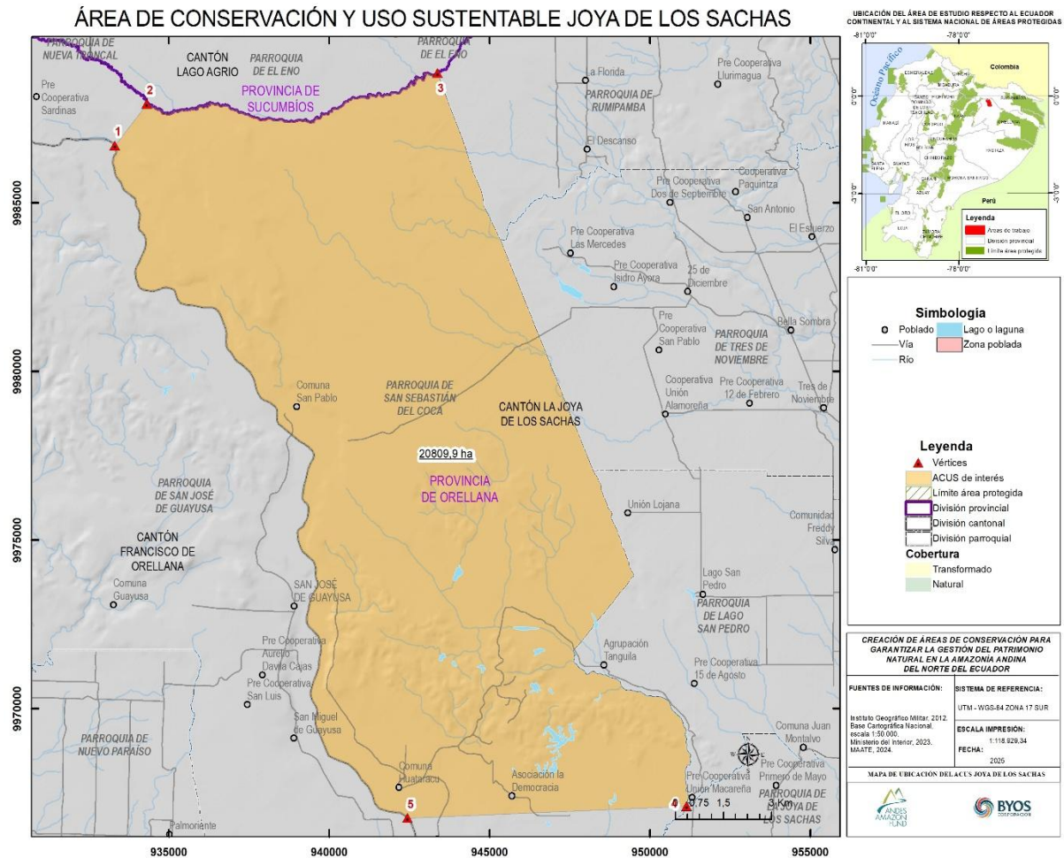
Figura 1. Mapa de ubicación y límites del “ACUS Municipal Joya de los Sachas”
