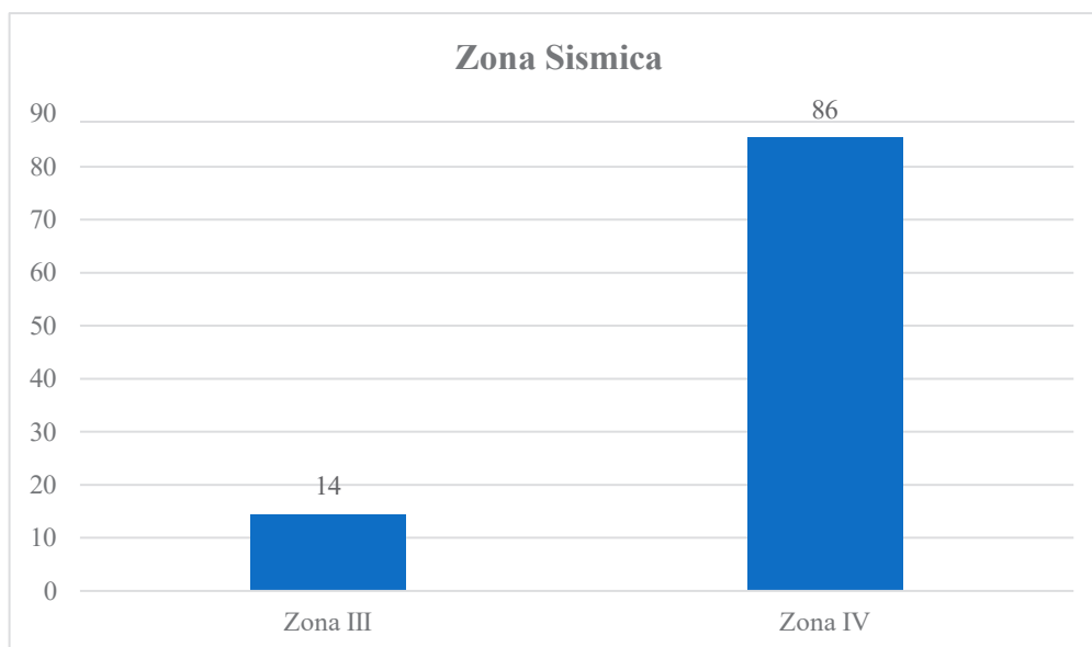
Ilustración 10: Zonas Sísmicas
