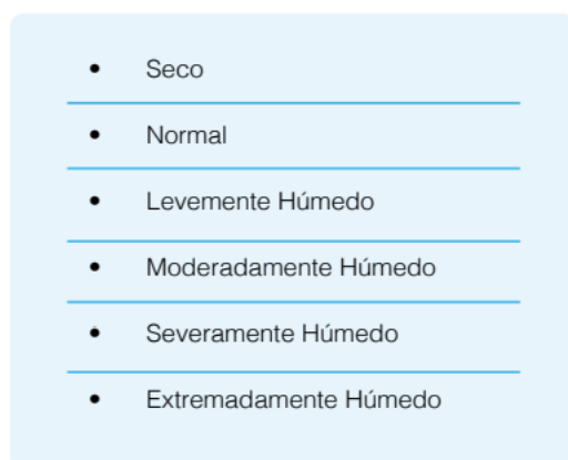
Gráfico No. 9: Índice de Precipitación y Evapotranspiración Estandarizado (SPEI)
