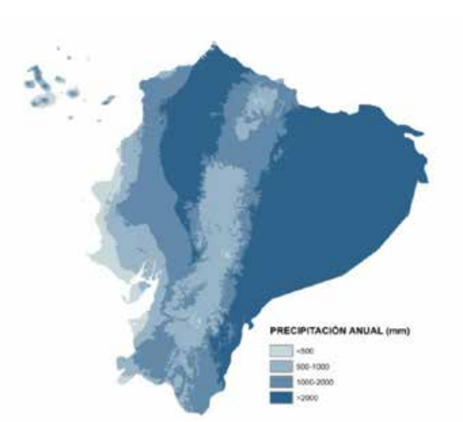
Mapa No. 20: Precipitación anual registrada en el Ecuador.
