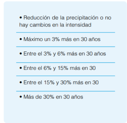
Gráfico No. 8: Índice de precipitación total
