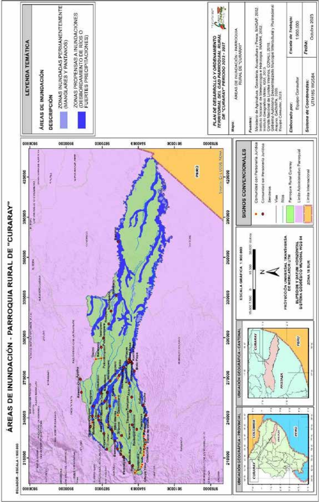
Mapa No. 15: Áreas de inundación en la parroquia Curaray
