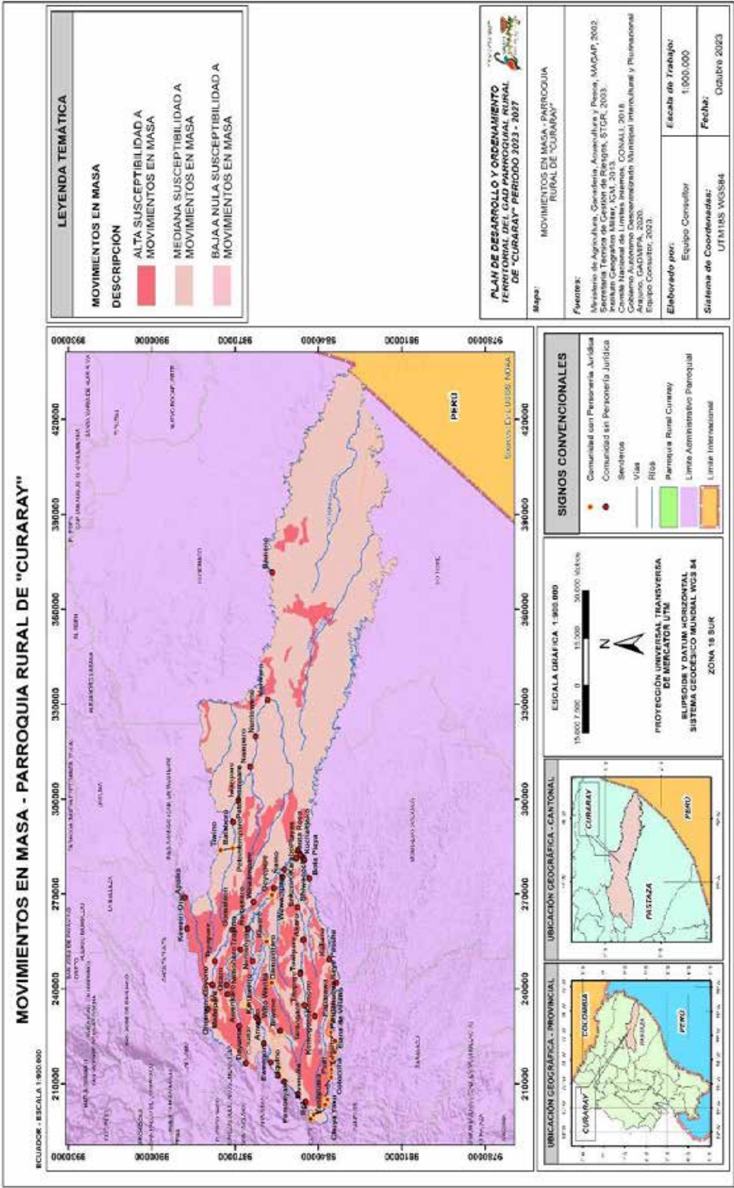
Mapa No. 13: Movimientos de masa en la parroquia Curaray
