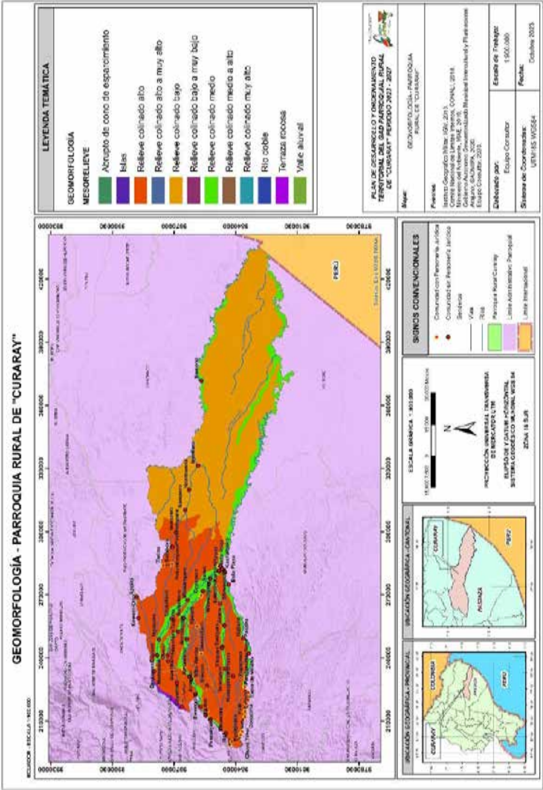
Mapa No. 7: Geomorfología de la parroquia Curaray
