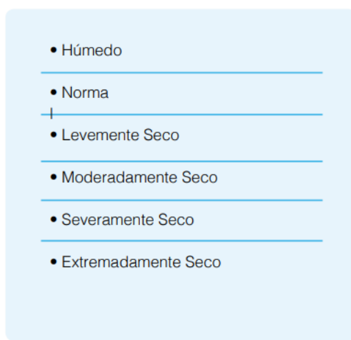
Gráfico No. 10: Índice de Condiciones de Sequedad se centra en las modificaciones de las transiciones entre las temporadas de mayores a menores lluvias, específicamente de húmedo a seca (SPEI)
