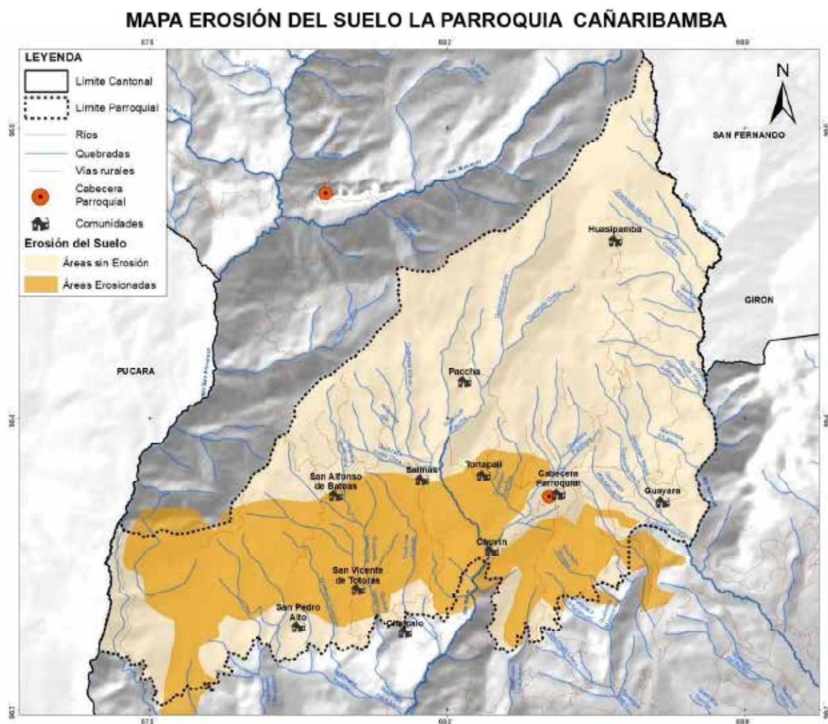
Figura 59. Mapa erosión de la Parroquia Cañaribamba Fuente: Ministerio del Ambiente, Agua y Transición Ecológica Elaboración: Equipo Consultor
