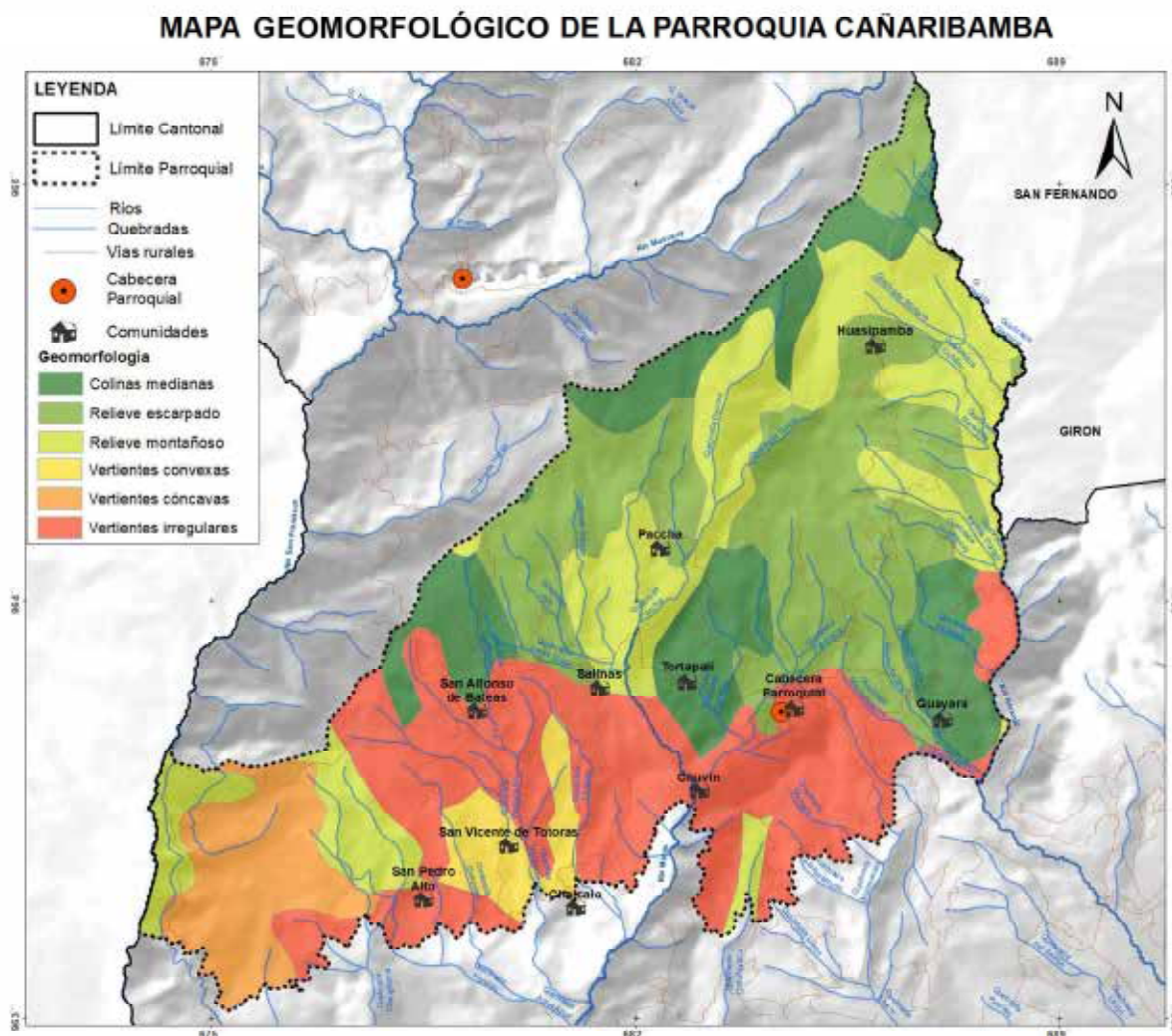
Figura 53. Mapa geomorfológico de la Parroquia Cañaribamba
