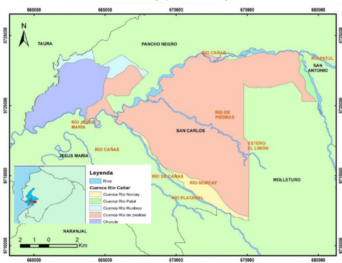
Ilustración 4: Hidrografía de la Parroquia San Carlos
