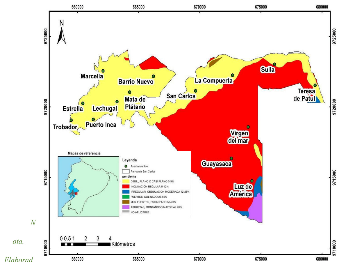
Ilustración 7 : Mapa de pendientes de la parroquia San Carlos
