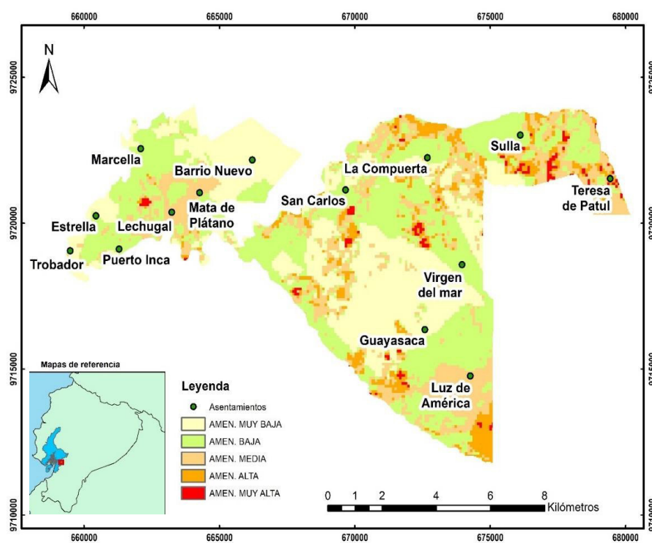
Ilustración 11: Mapa de amenaza de movimientos en masa
