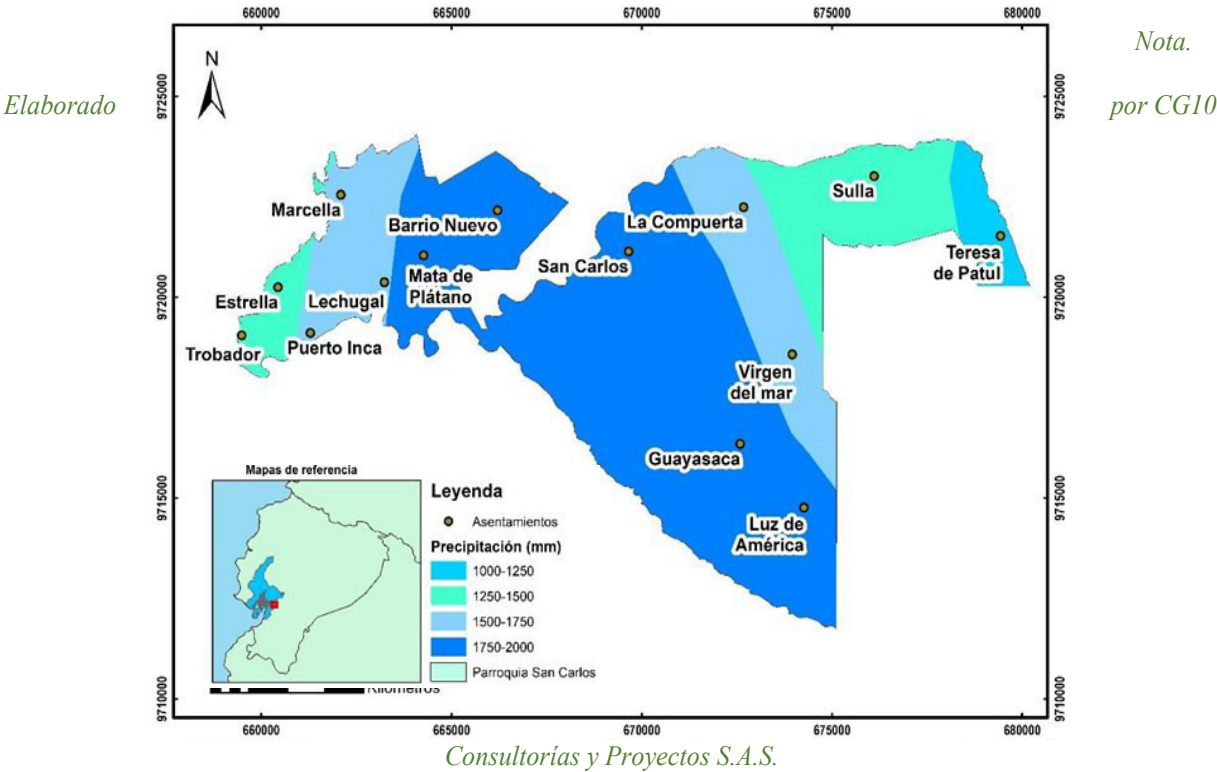
Ilustración 14: Mapa de Isoyetas de la parroquia San Carlos
