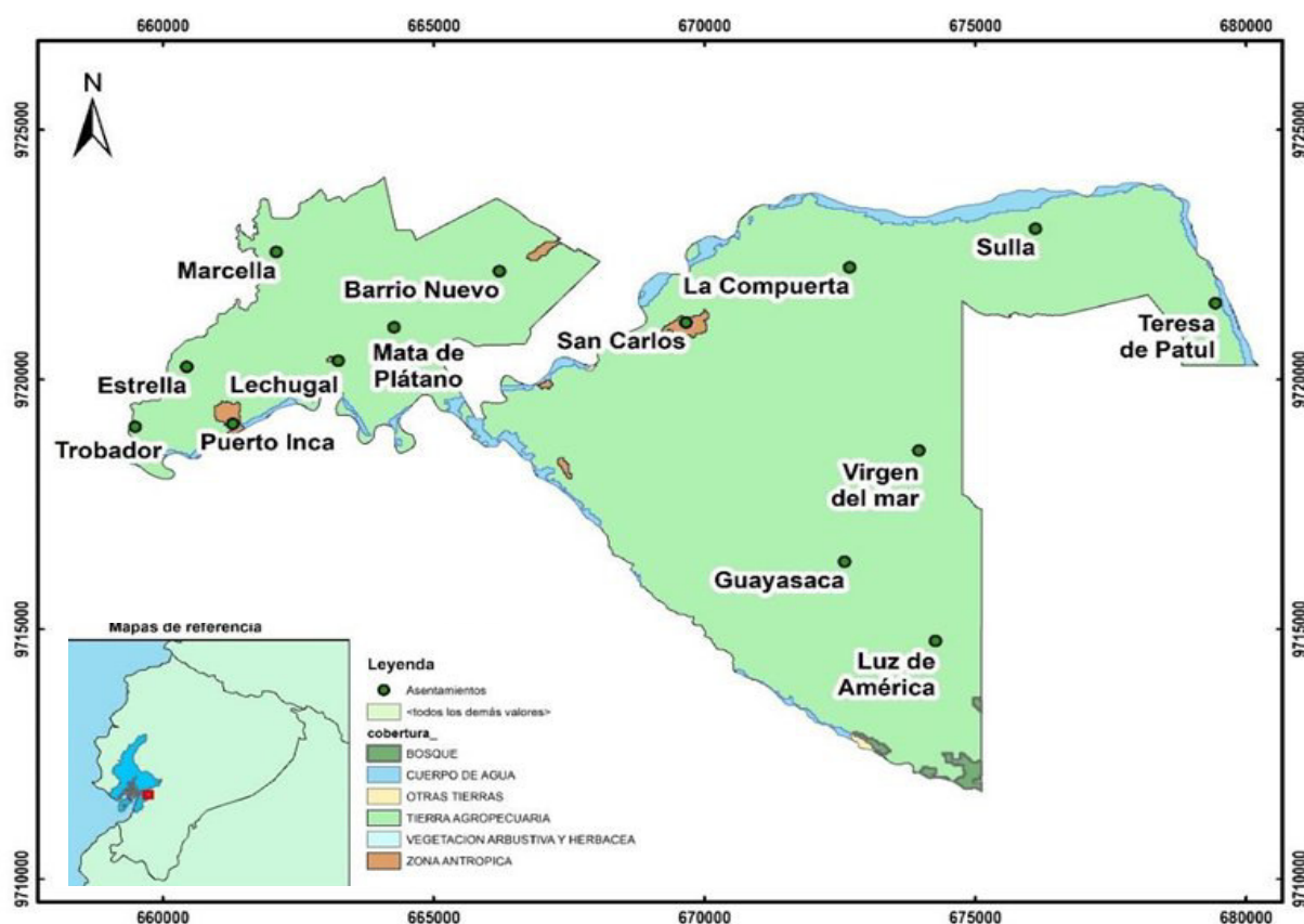
Ilustración 9: Mapa de cobertura del suelo
