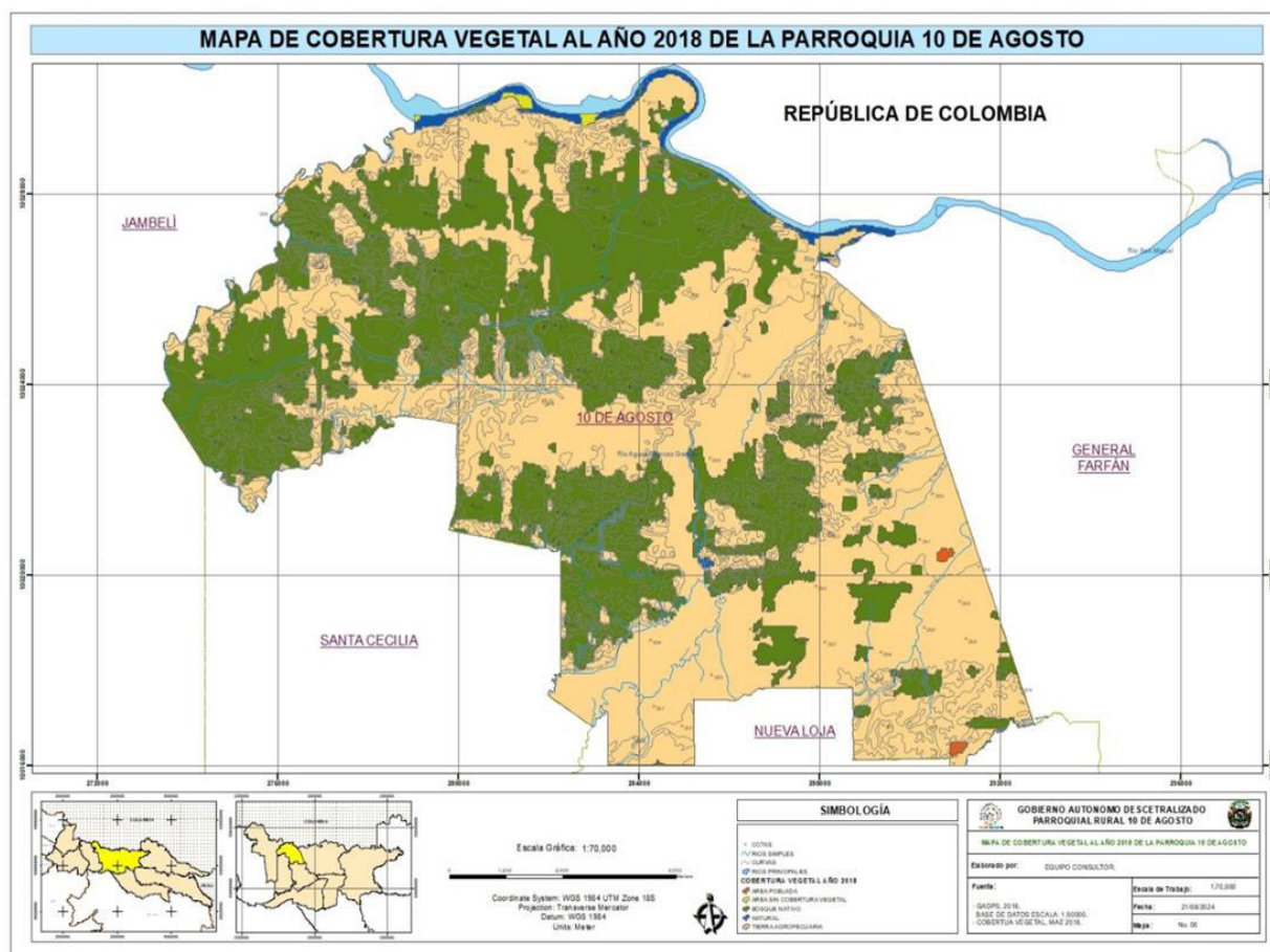
Figura 17. Cobertura vegetal, uso y ocupación del suelo
