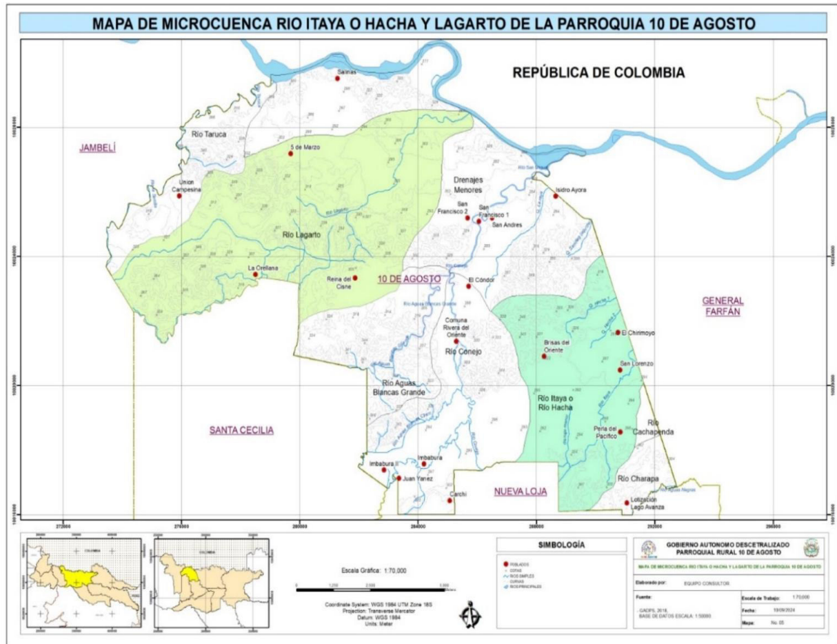
Figura 14. Microcuencas de los ríos Hacha y Lagarto
