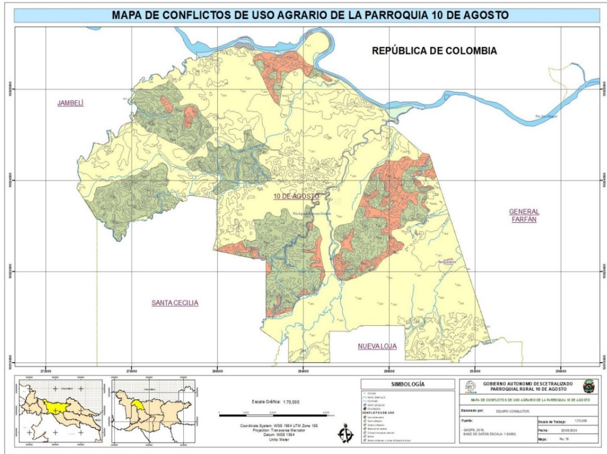
Figura 13. Conflicto de uso del suelo
