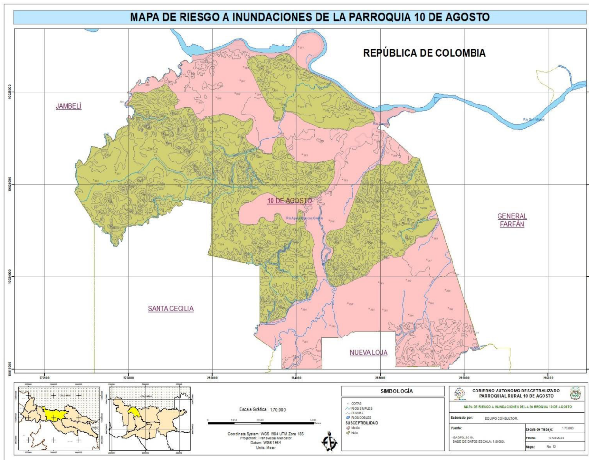
Figura 10. Territorio susceptible a inundaciones
