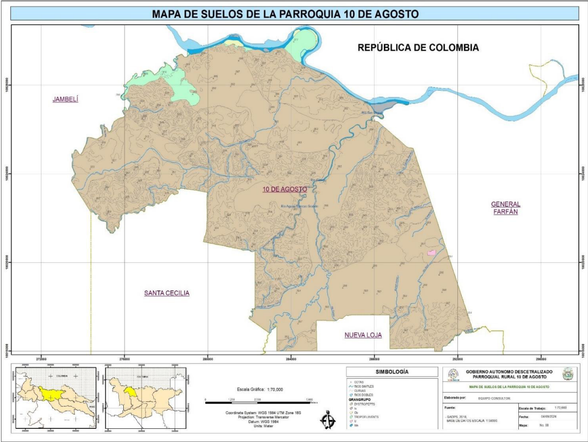
Figura 6. Tipos de suelo
