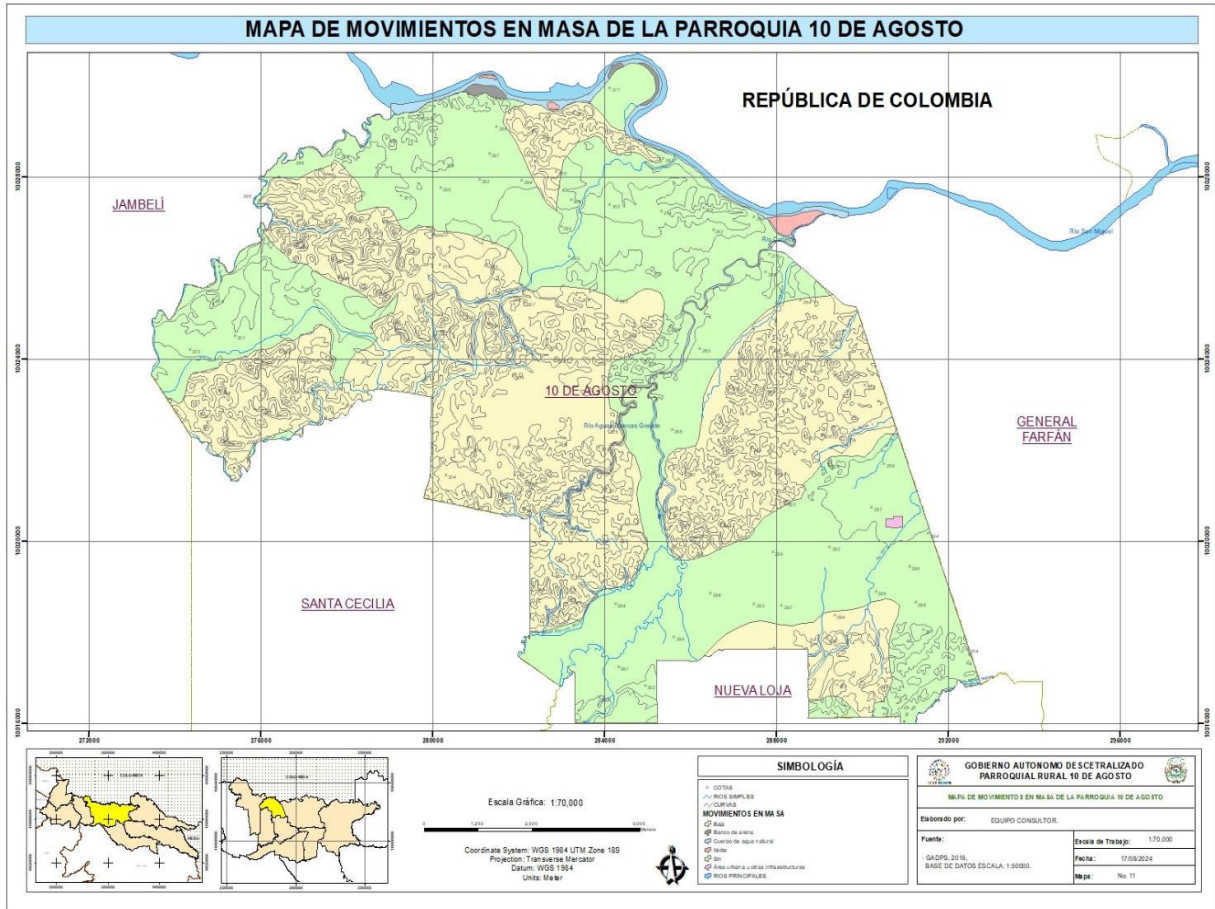
Figura 9. Territorio, susceptible a movimientos en masa
