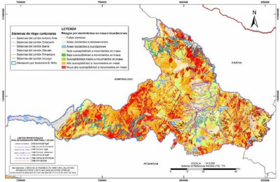
Mapa 42. Sistemas de riego vulnerables a deslizamientos en Imbabura.
