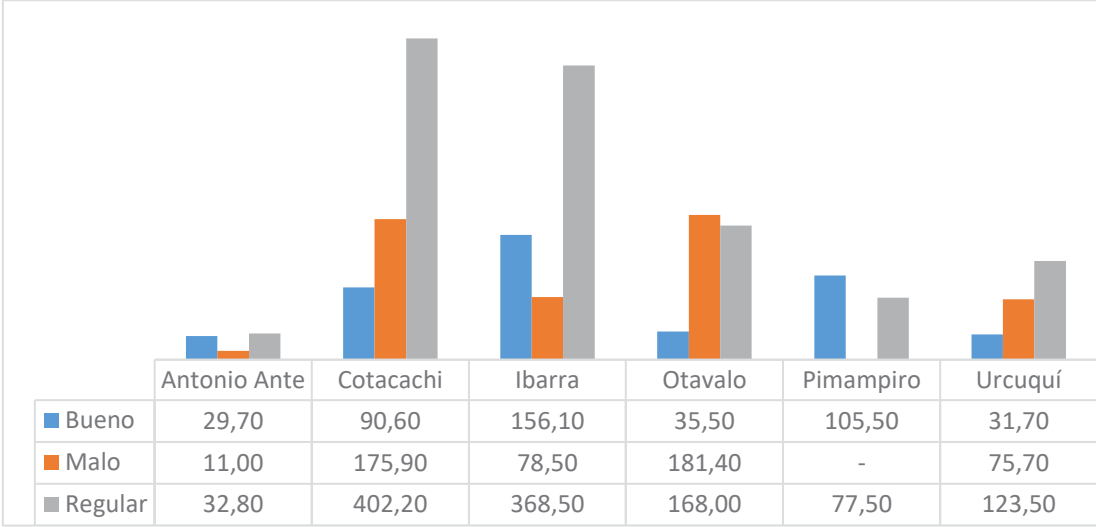
Figura 104. Estado de la capa de rodadura (km).
