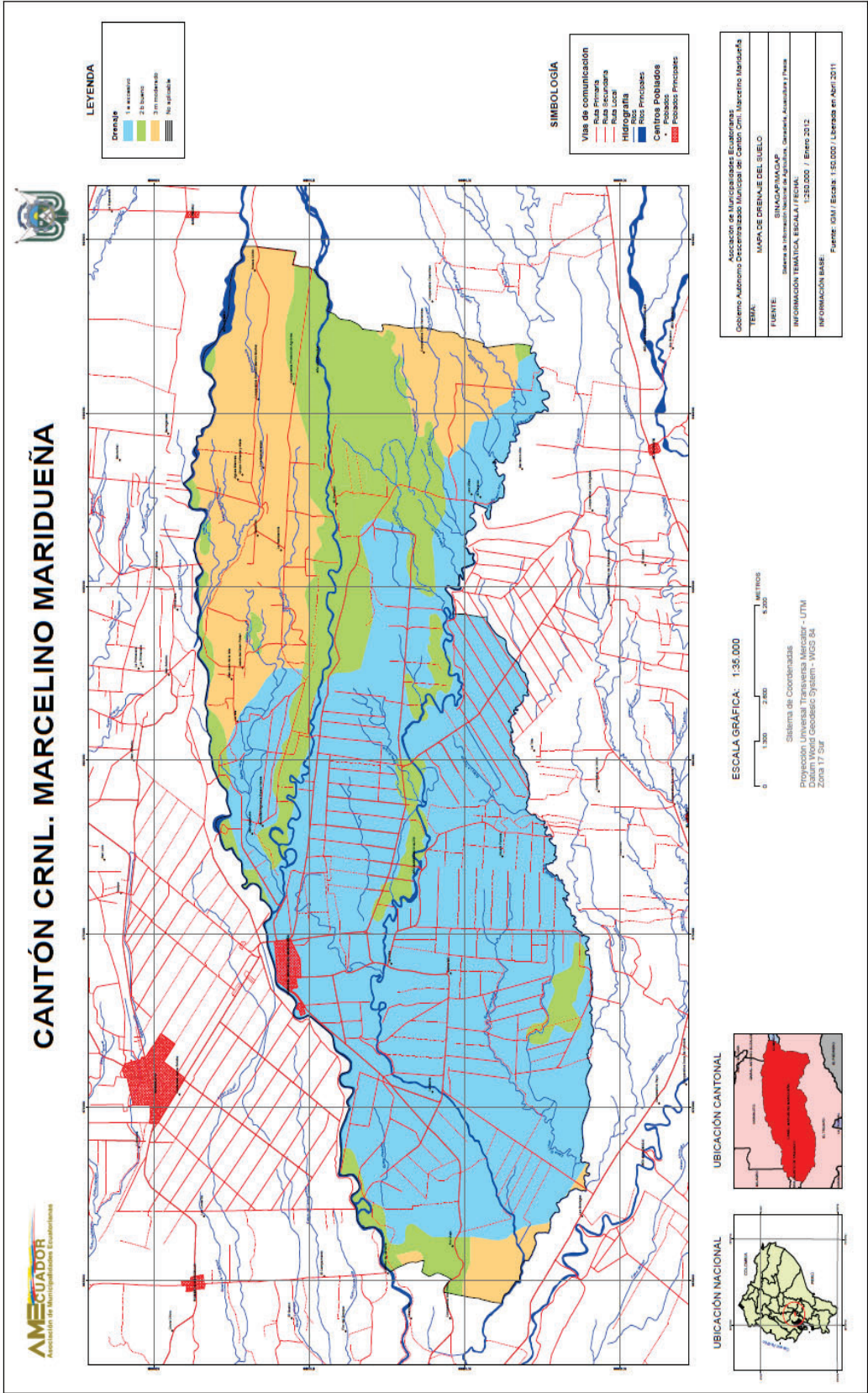
MAPA # 5.- DRENAJE
