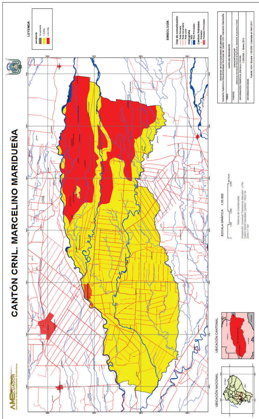
MAPA# 3.- PENDIENTE
