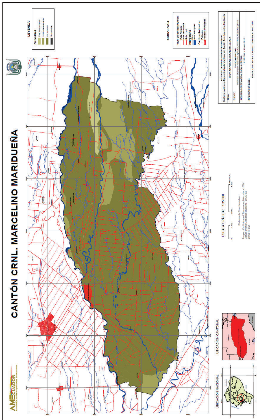
MAPA # 4.- PROFUNDIDAD
