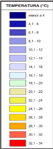
Ilustración 3. Temperatura media anual observada en el periodo histórico 1981-2015, en la Provincia de Manabí.
