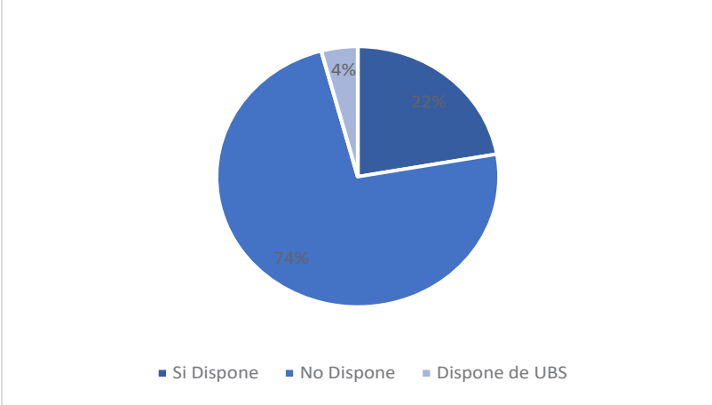
Gráfico 40 Disponibilidad de Sistemas de Alcantarillado en los poblados del Cantón.
