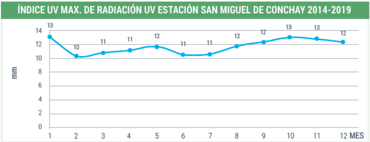
Gráfico 5 Índice max. De radiación uv estación San Miguel de Conchay 2014-2019
