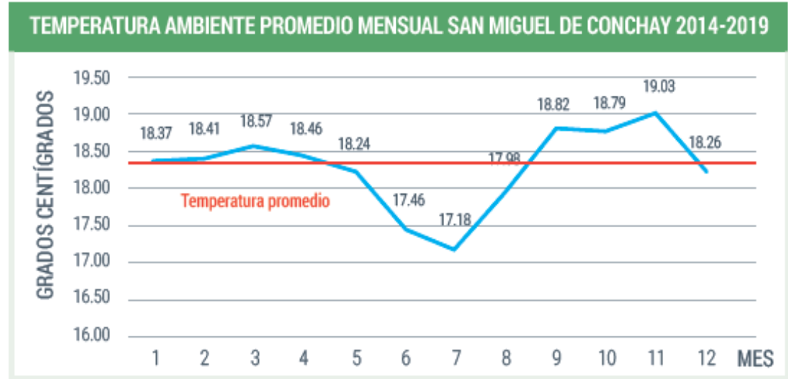
Gráfico 3 Temperatura ambiente promedio mensual San Miguel de Conchay (2014-2019)
