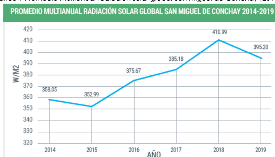
Gráfico 9 Promedio multianual radiación solar global San Miguel de Conchay (2014-2019)
